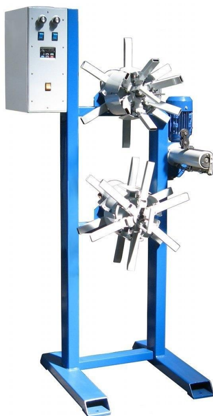
Рис.1 Общий вид бухтонамотчика.
